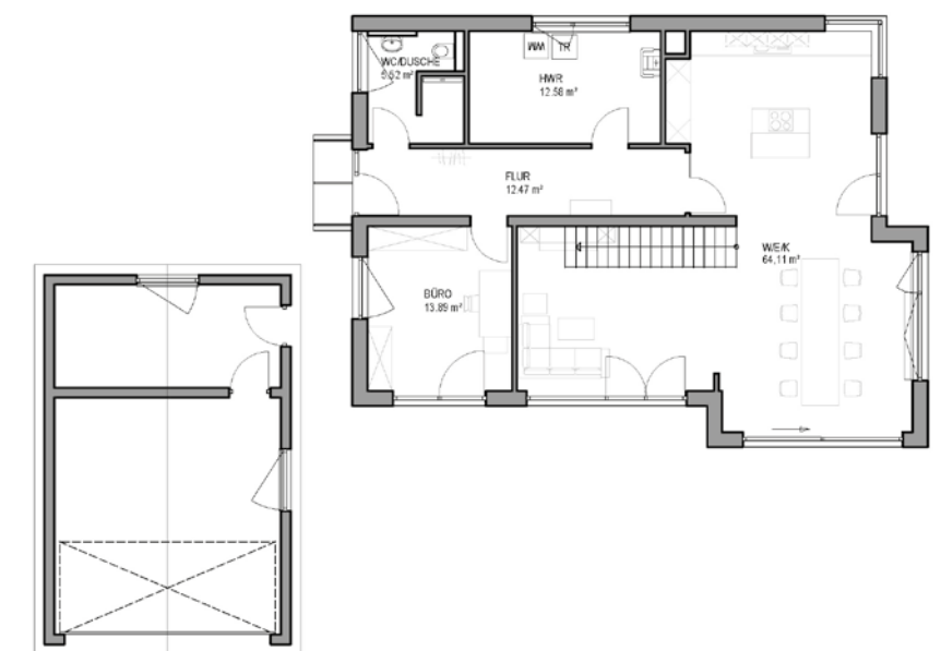
Grundriss EG
