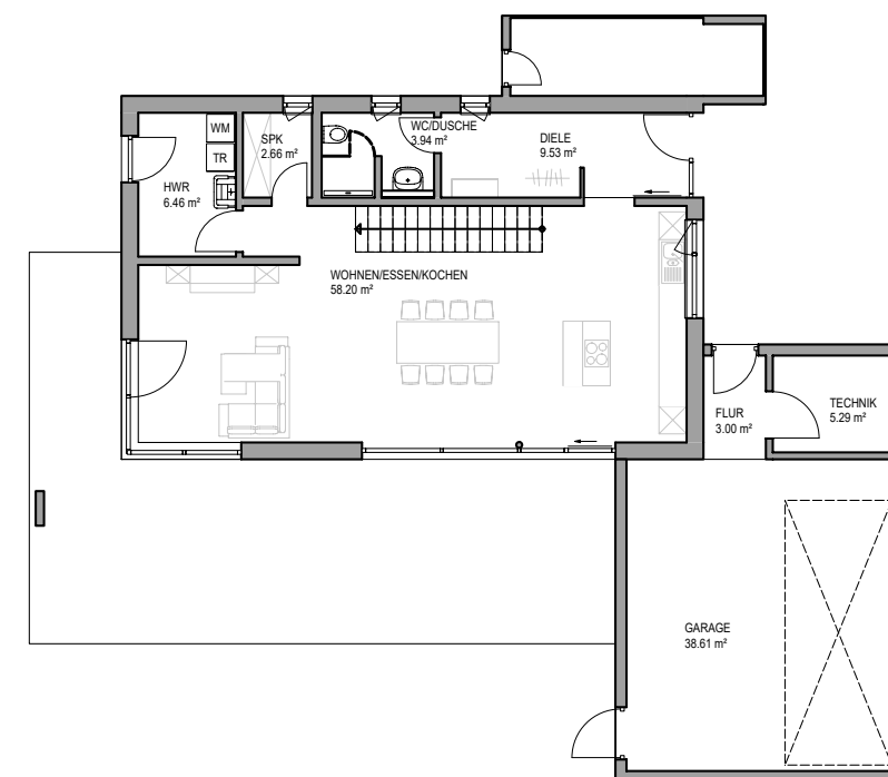
Grundriss EG
